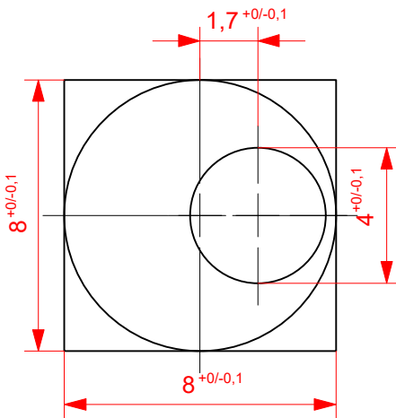
detail A schaal 1:5
